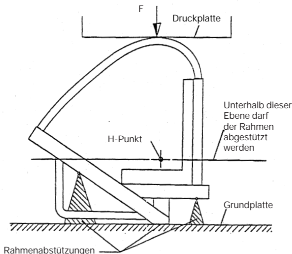
Versuchsaufbau Dachdrückttest
