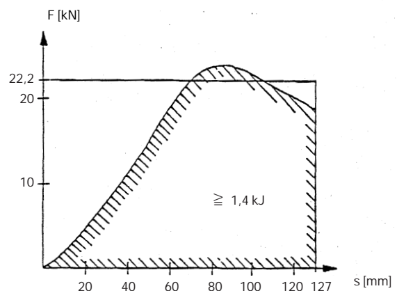
Kraft-Weg-Diagramm Dachdrückttest
