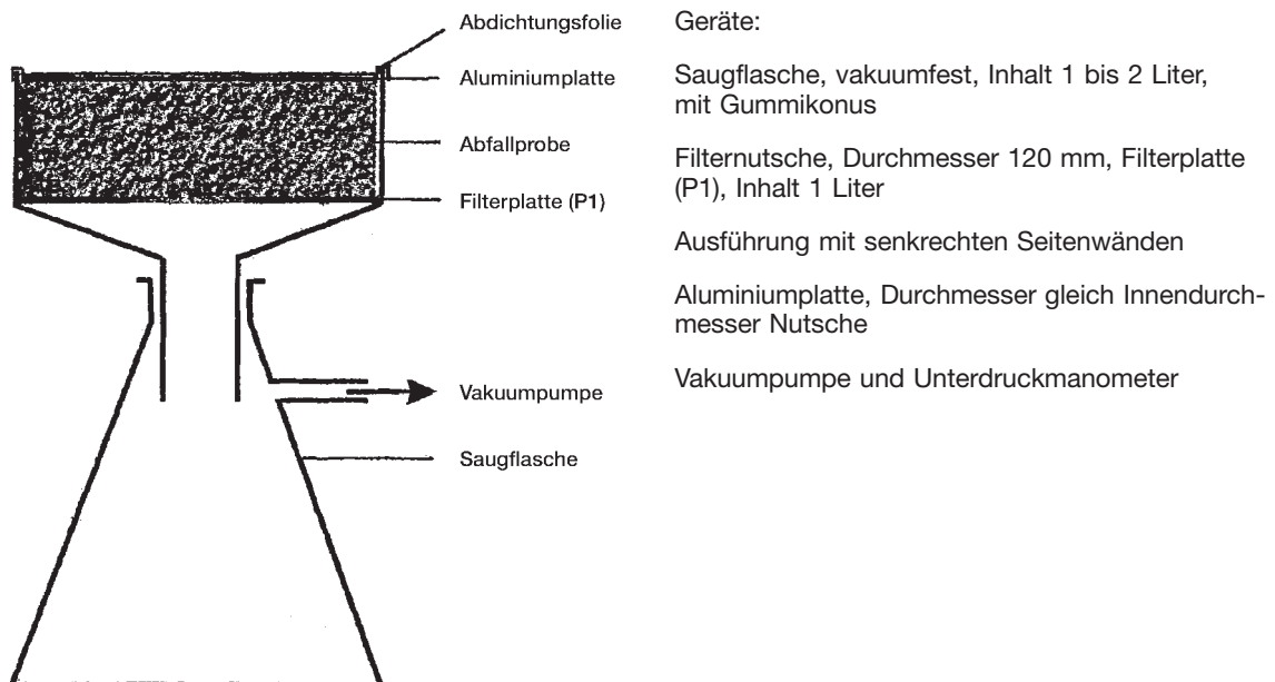
Bild 1: Apparatur zur Einstellung des Wassergehaltes
