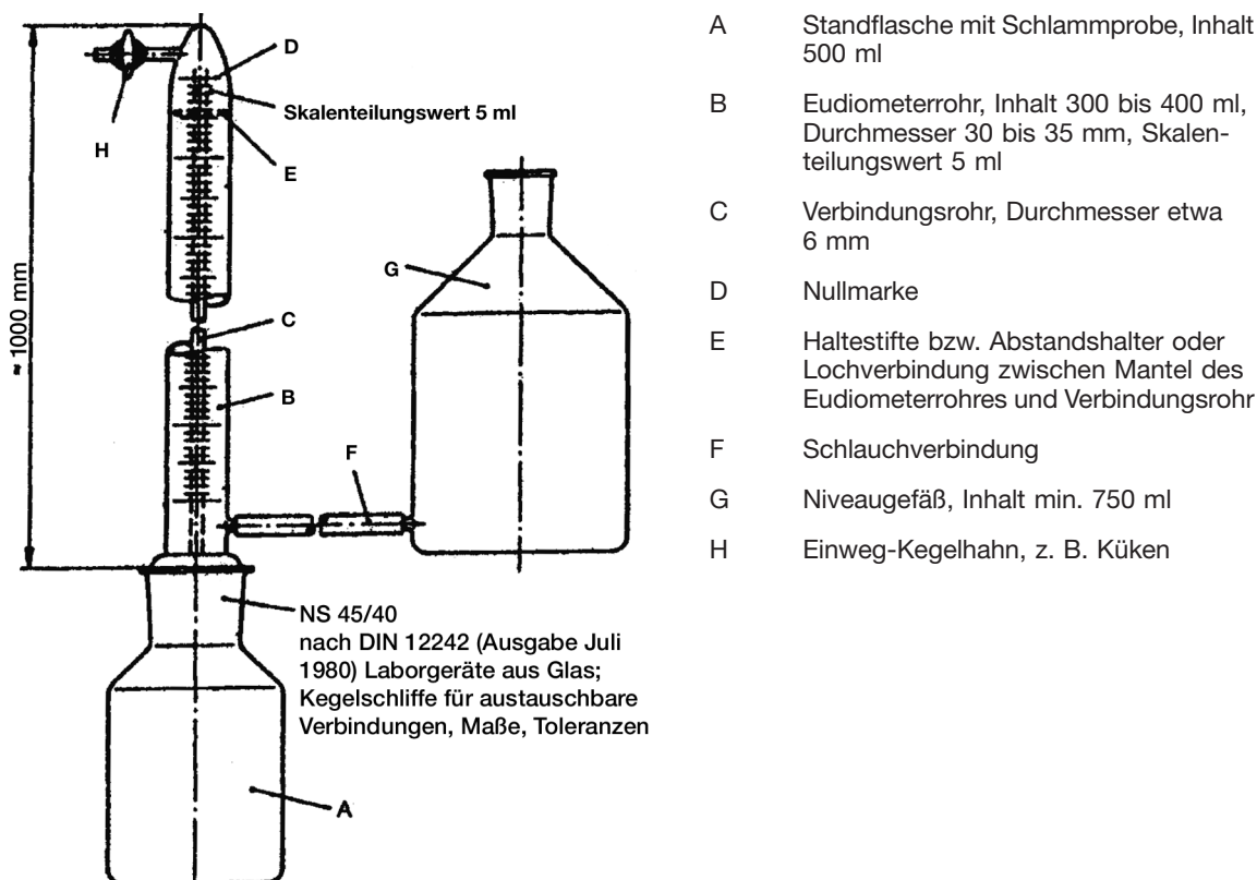
Bild 2: Versuchsanordnung zur Bestimmung des Faulverhaltens von Schlamm nach DIN 38414-8, Seite 6, Ausgabe Juni 1985
