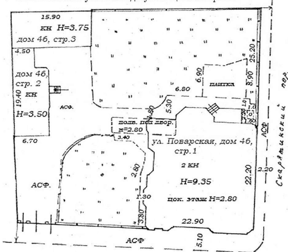
План земельного участка по документации МосгорБТИ.
