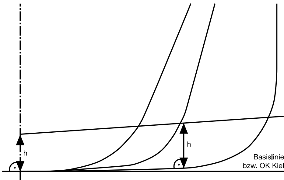
Abb. 3 – Begrenzungslinien des Ladetanks im Sinne des Absatzes 6
