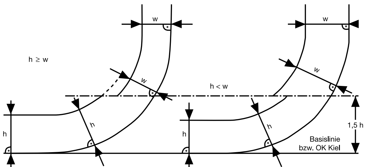
Abb. 1 – Begrenzungslinien des Ladetanks im Sinne des Absatzes 3
