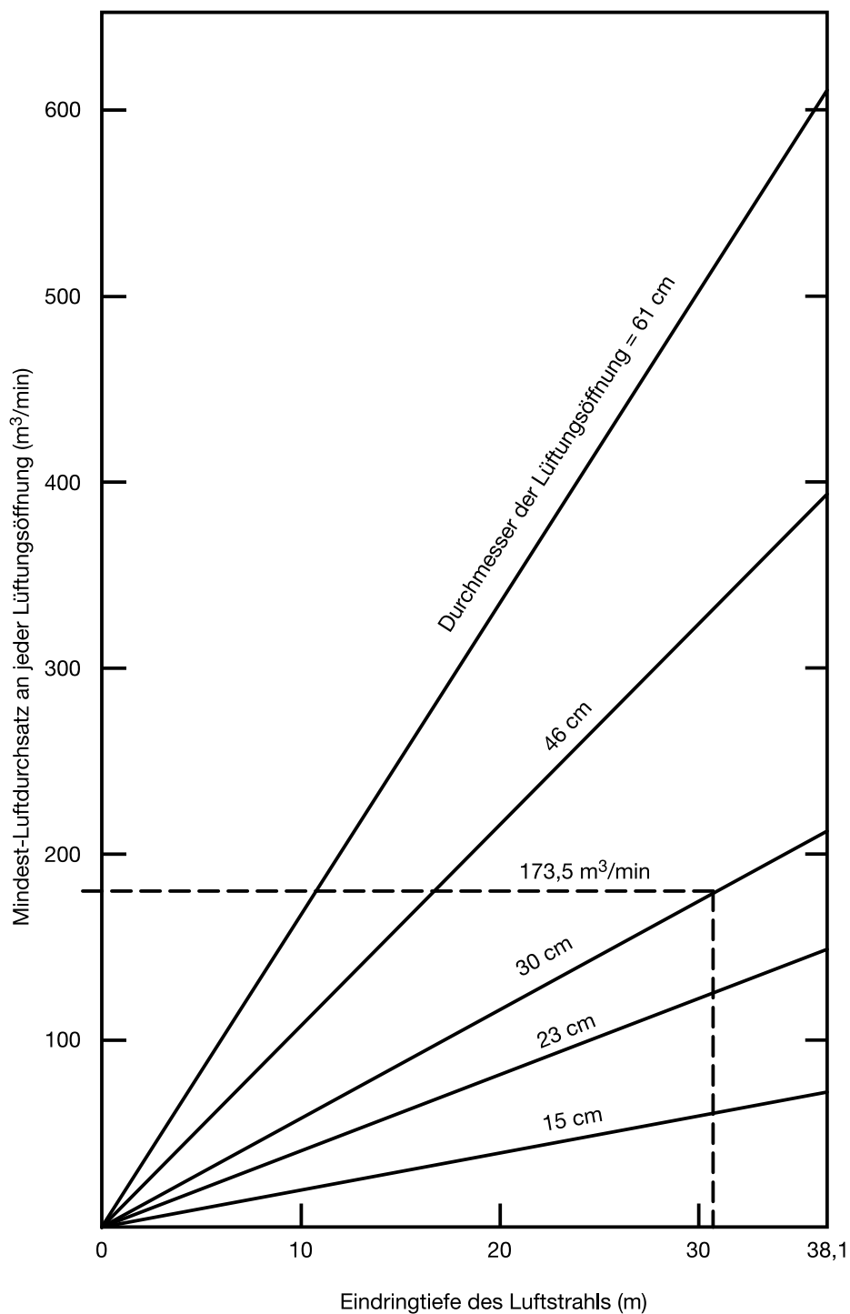
Abbildung 7-1. Mindest-Luftdurchsatz in Abhängigkeit von der Eindringtiefe des Luftstrahls. Die Eindringtiefe des Luftstrahls ist mit der Höhe der Tankwand zu vergleichen.
