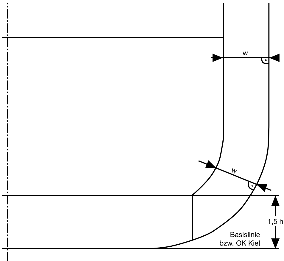
Abb. 2 – Begrenzungslinien des Ladetanks im Sinne des Absatzes 4
