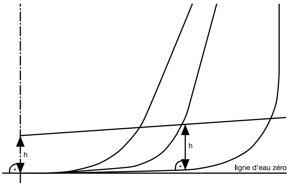
Figure 3 – Limites des citernes à cargaison aux fins du paragraphe 5
