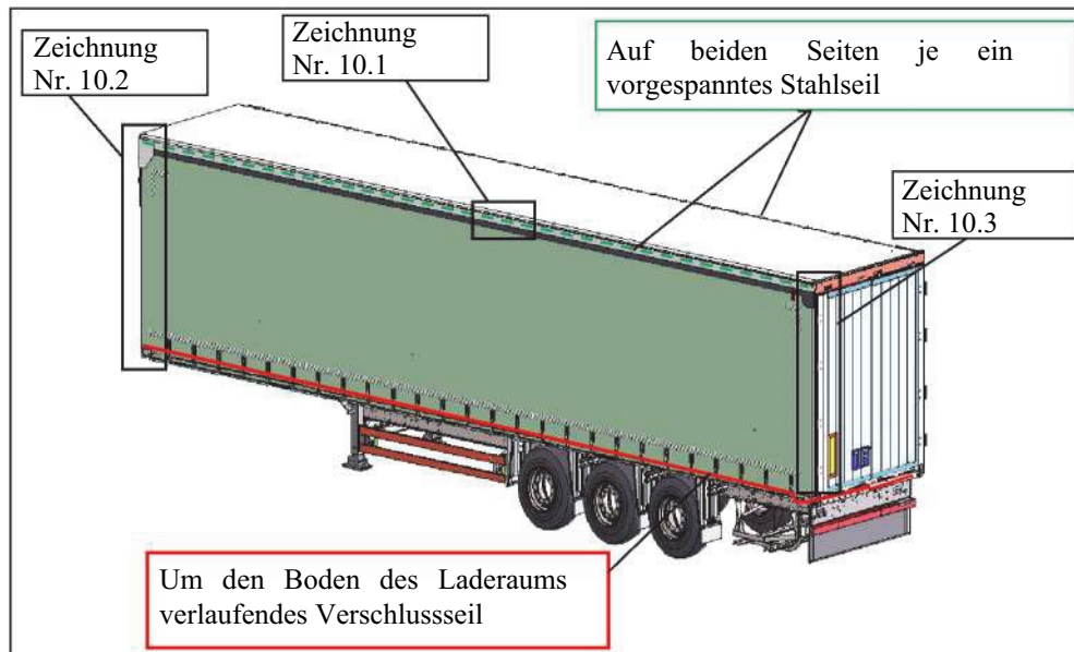
Zeichnung Nr. 10.1
