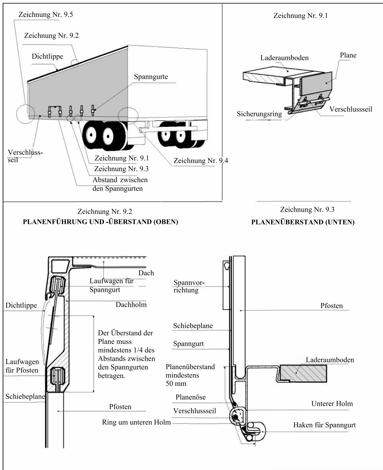
Zeichnung Nr. 9
