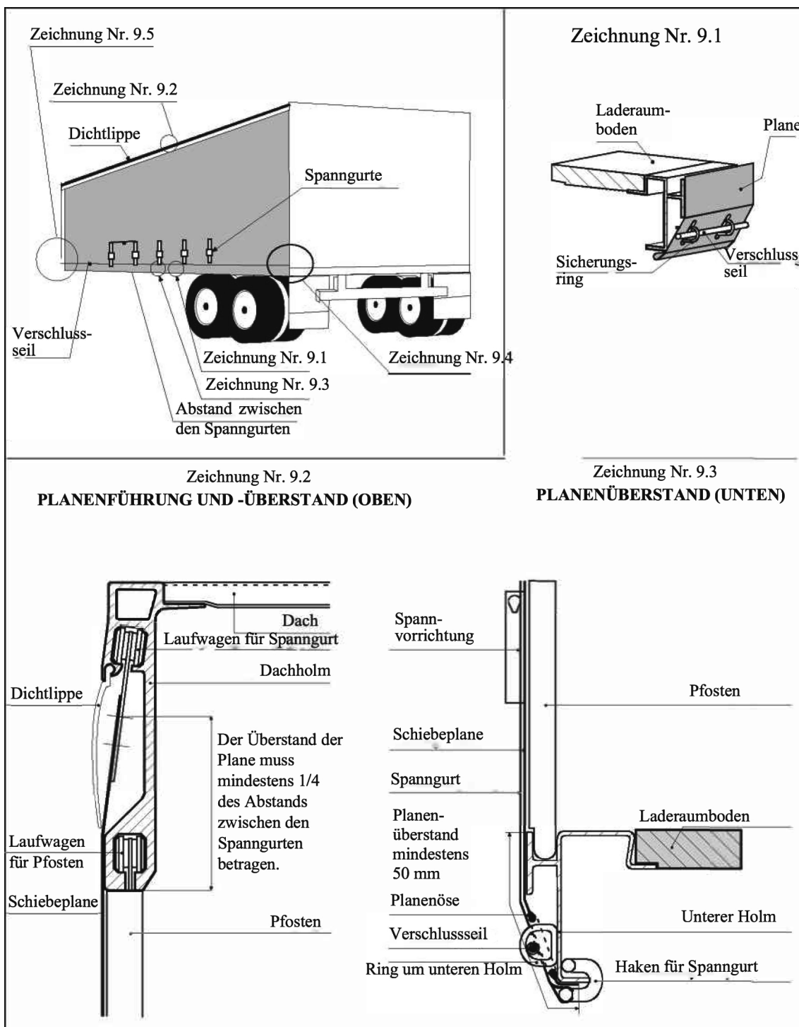
Zeichnung Nr. 9
